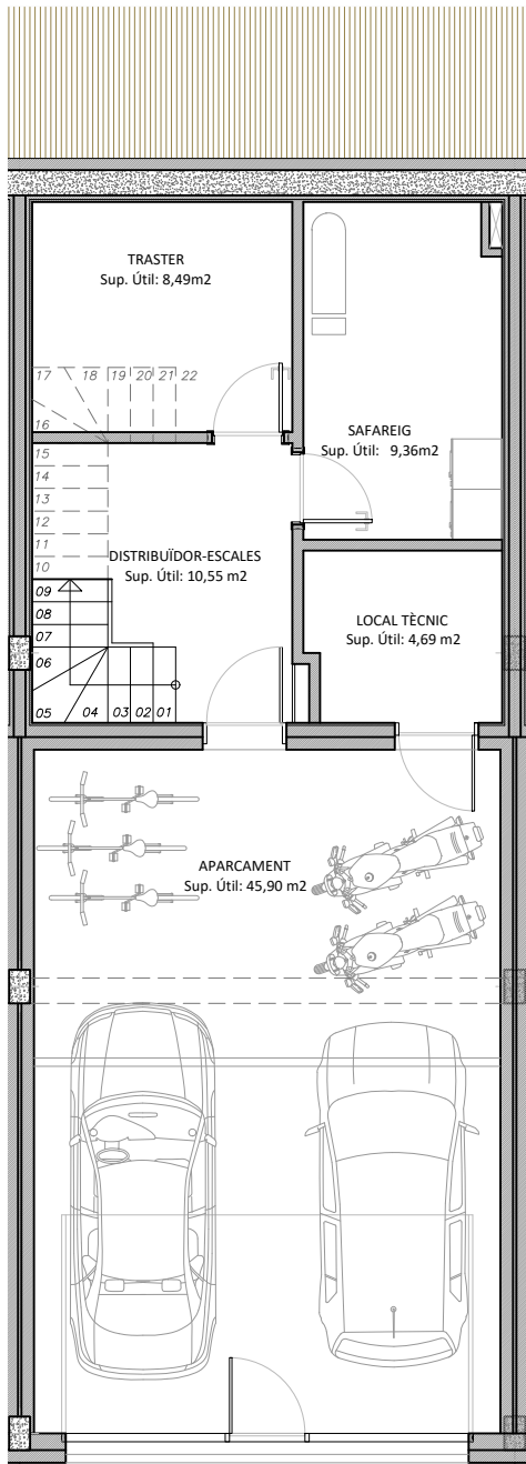
PLANTA SOTERRANI
