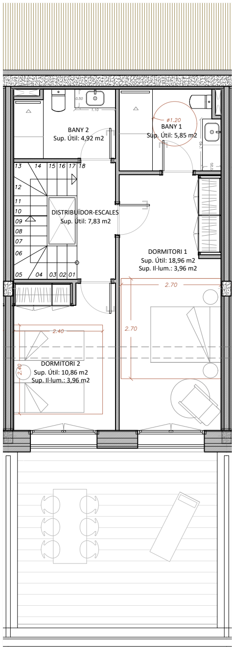
PLANTA PRIMERA
