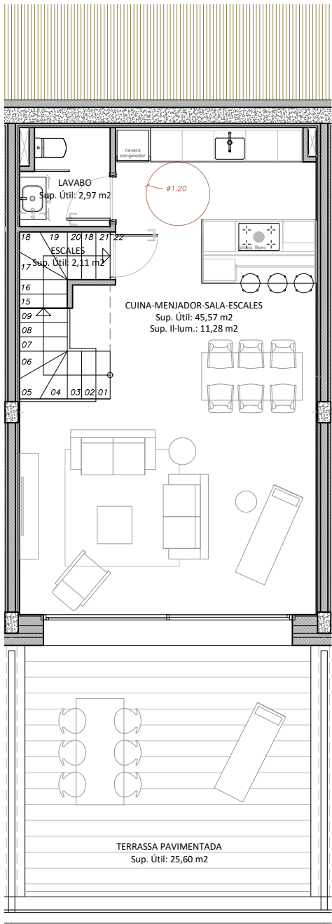
PLANTA BAIXA
