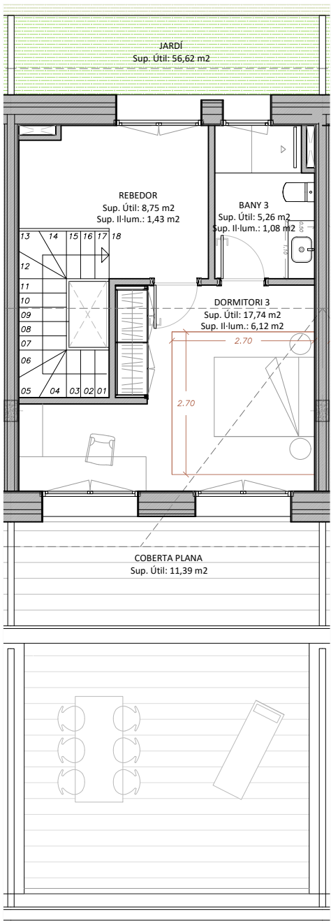
PLANTA SOTACOBERTA
